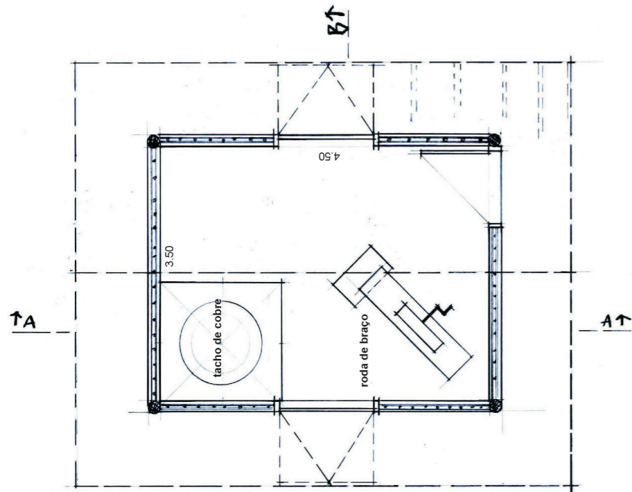
PLANTA esc. 1/75
