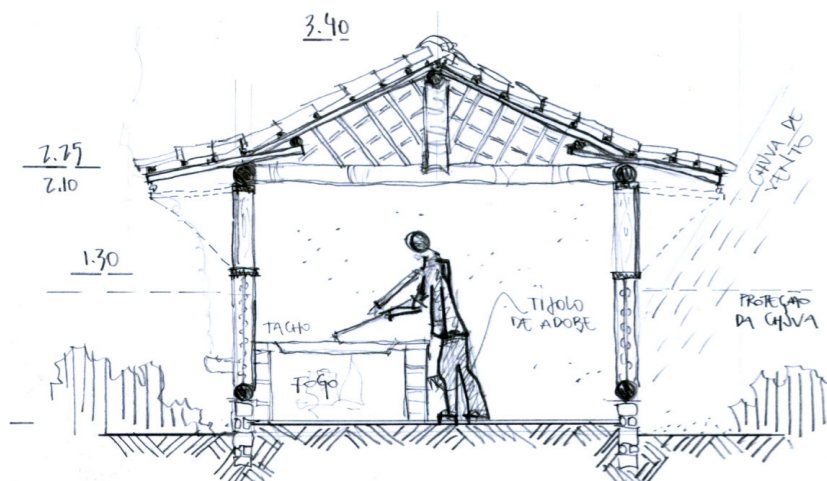
CORTE BB esc. 1/75
